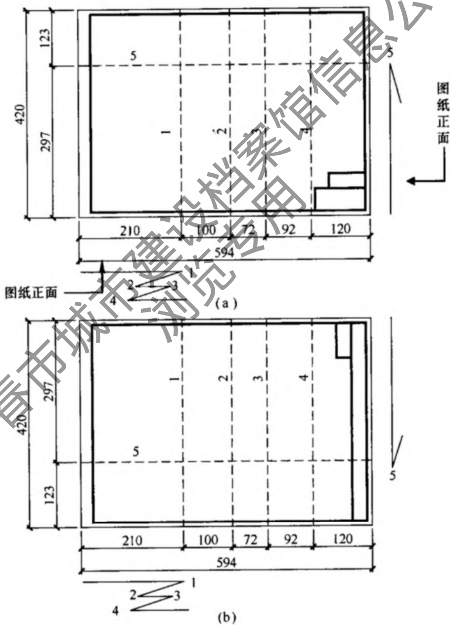
E. 0. 2-2 2# 图纸折叠示意
